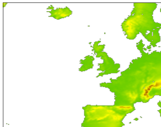
(b) WRF 18 km
