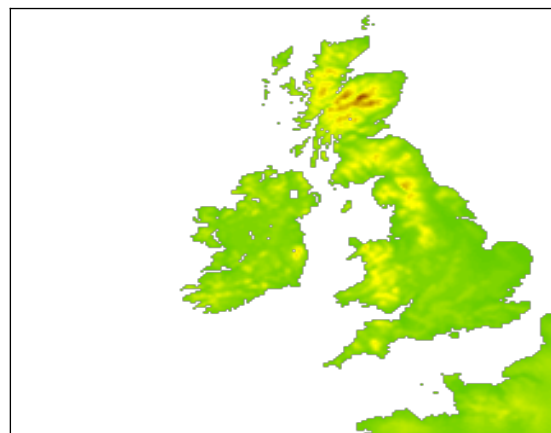
(d) WRF 6 km
