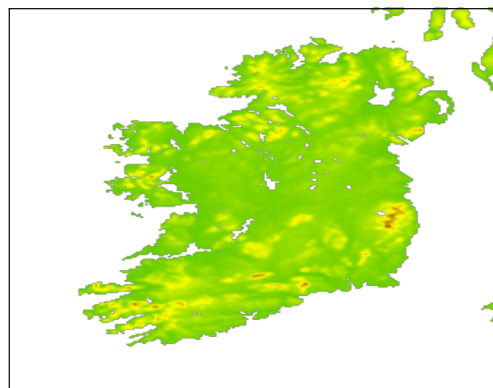
(f) WRF 2 km
